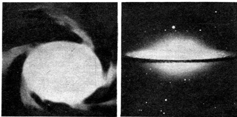
A g. : La plus célèbre photo de soucoupe (1952, Baléares). Celle-ci peut provenir d'une de ces nébuleuses d'étoiles (à dr.) dont la lumière, à la vitesse de 300.000 km-seconde met des millions d'années à nous parvenir.
